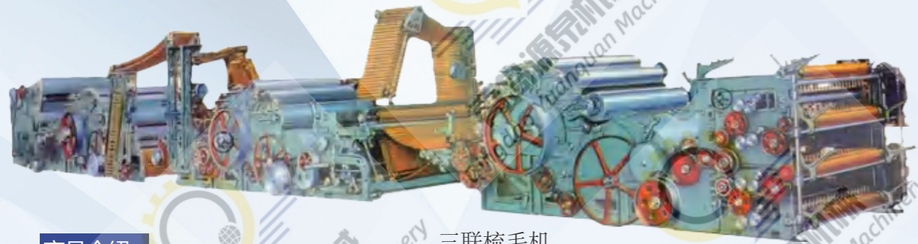
三联梳毛机 Triple-Component
